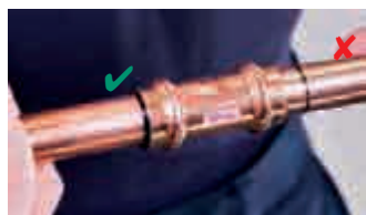
8. Insérez complètement le tube dans le raccord. Assurez-vous que le tube soit complètement inséré avant sertissage
